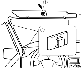
① مشبك الميكروفون ② مشابك
